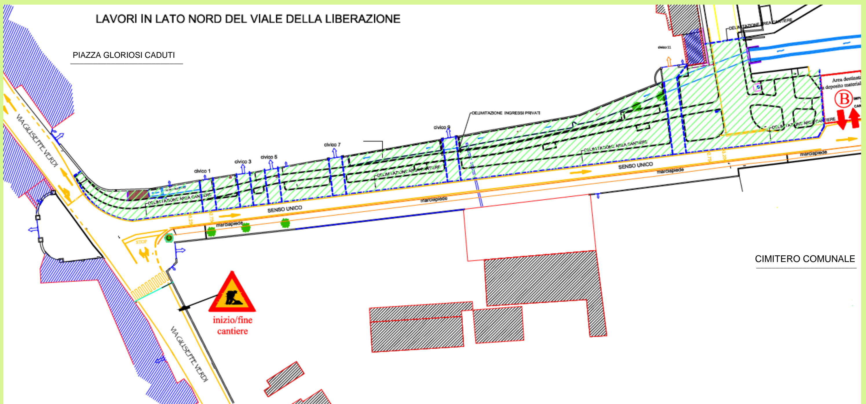
FASE 1 - LAVORAZIONI IN LATO NORD DEL VIALE LIBERAZIONE ISTITUZIONE SENZO UNICO IN DIREZIONE USCITA DAL PAESE
